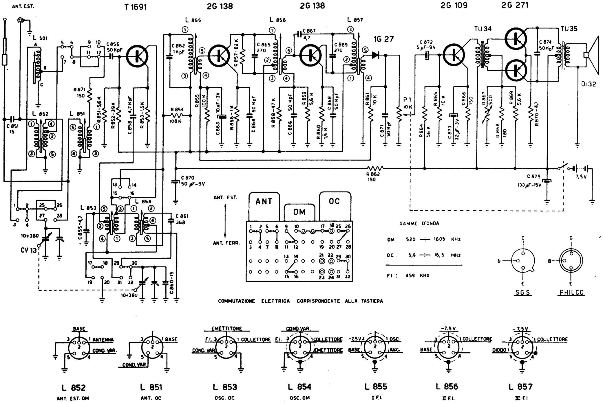
Schema elettrico del radoricevitore MAGNADYNE Mod. MD6041
